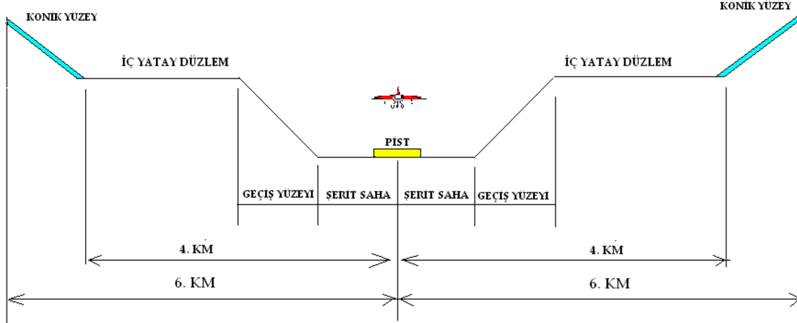
Şekil 5. (devam) Konik Yüzey Kesiti Gösterimleri
