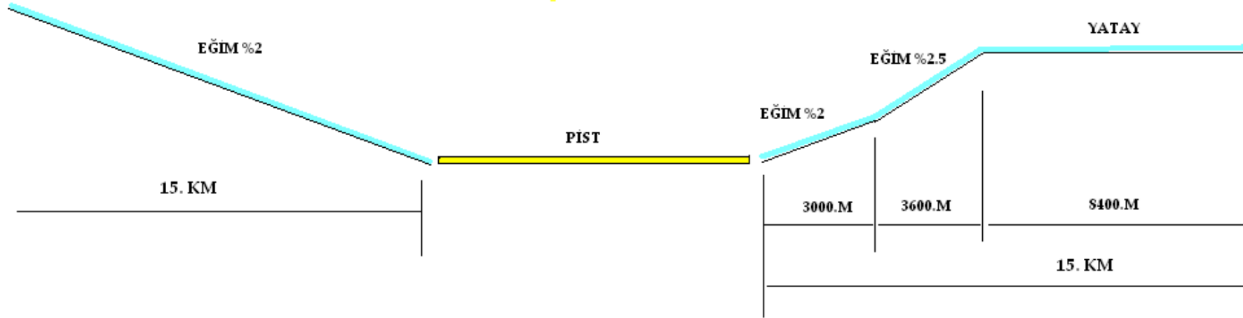
Şekil 3. Yaklaşma, Kalkış-Tırmanış Yüzey Gösterimleri
