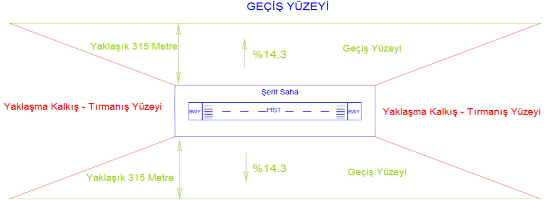
Şekil 2. Geçiş Yüzeyi Gösterimleri
